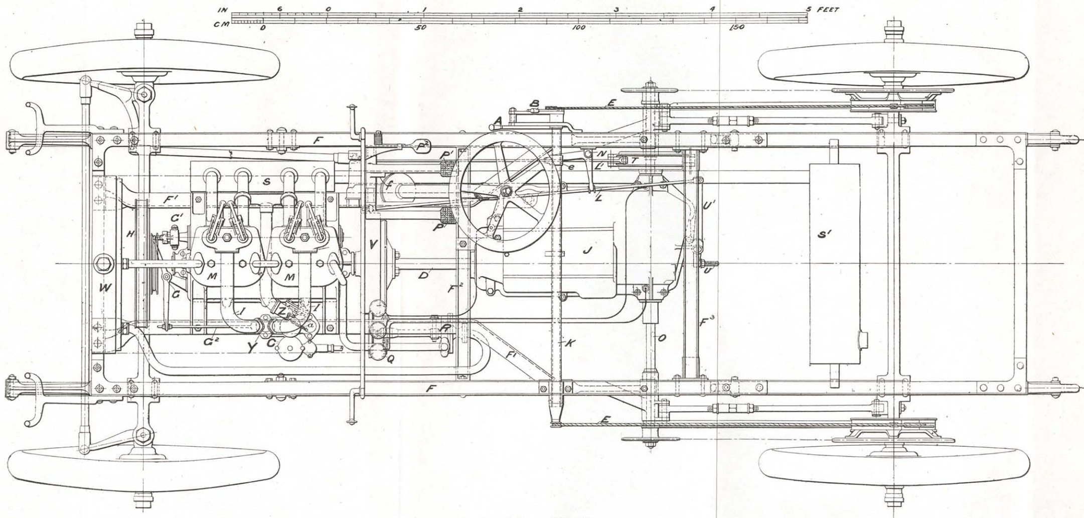
FIG. 256.—15-HP. NAPIER.
