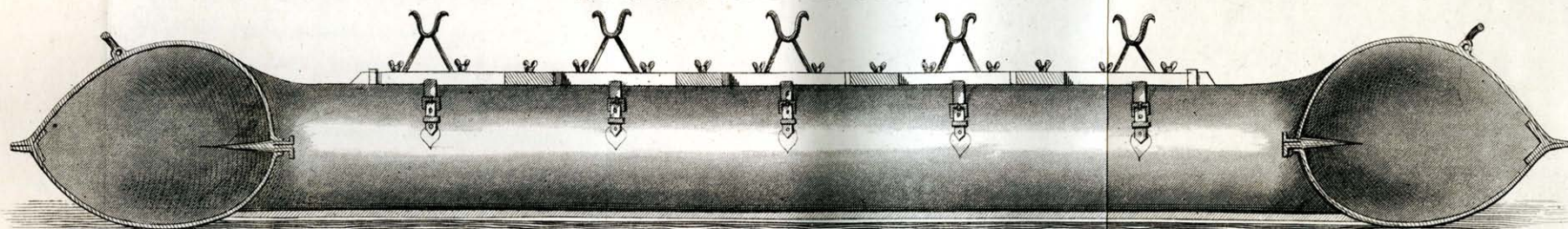
LONGITUDINAL SECTION.
