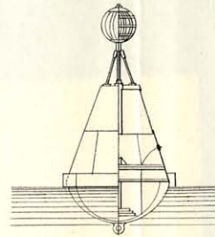
Fig. 14. BEACON BUOY.
