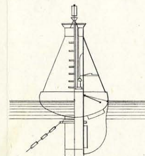
Fig. 17. WHISTLING BUOY.
