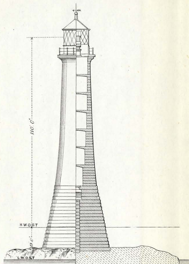
Fig. 3. WOLF ROCK.
