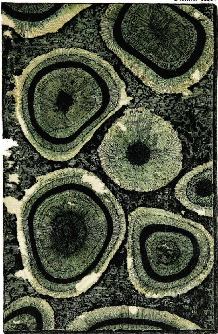
Granit Orbiculaire de Corse.
