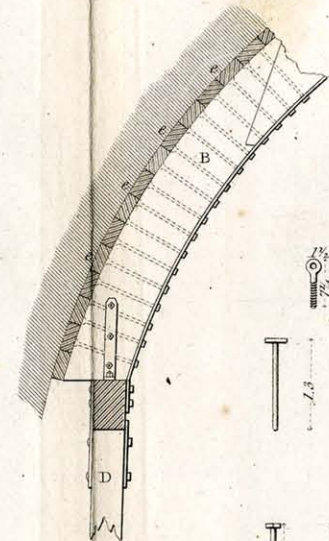
Fig. 7. Middle Rib
